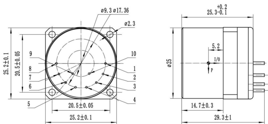
方形法兰尺寸
