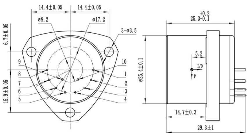
图一：标准版加速度计
