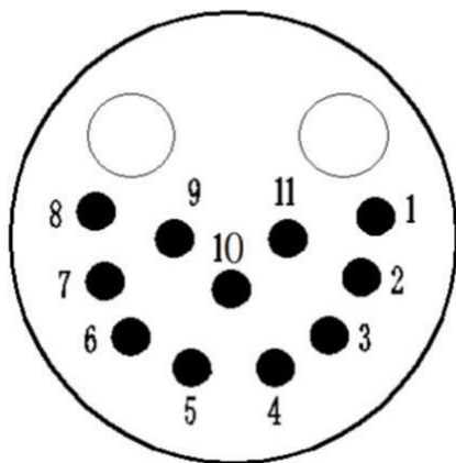
图 1 接线定义 (标准型)
